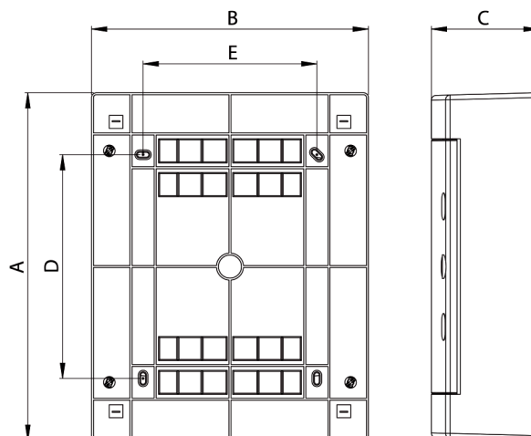
Obudowy natynkowe ECT
