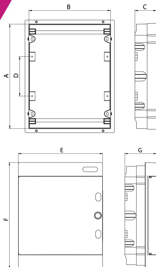
Obudowy podtynkowe ECM
