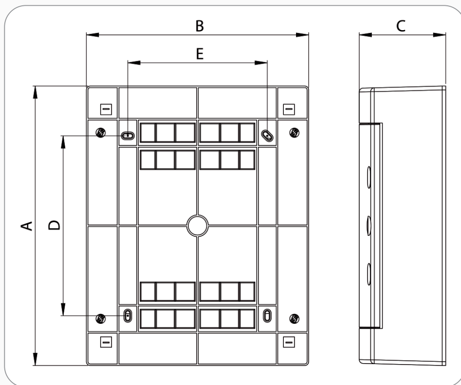
Obudowy natynkowe ECT
