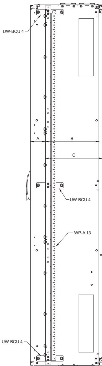
Obudowa z uchwytami UW-BCU 4 do wsporników pionowych WP-A
