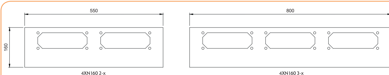
Otwór przepustu-standard C(FL 21)
