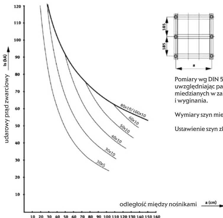
Wytrzymałość zwarciova w zależności od odległości między nośnikami (rozstaw szyn 185 mm)
