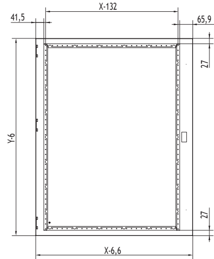
Zamek 3-punktowy
