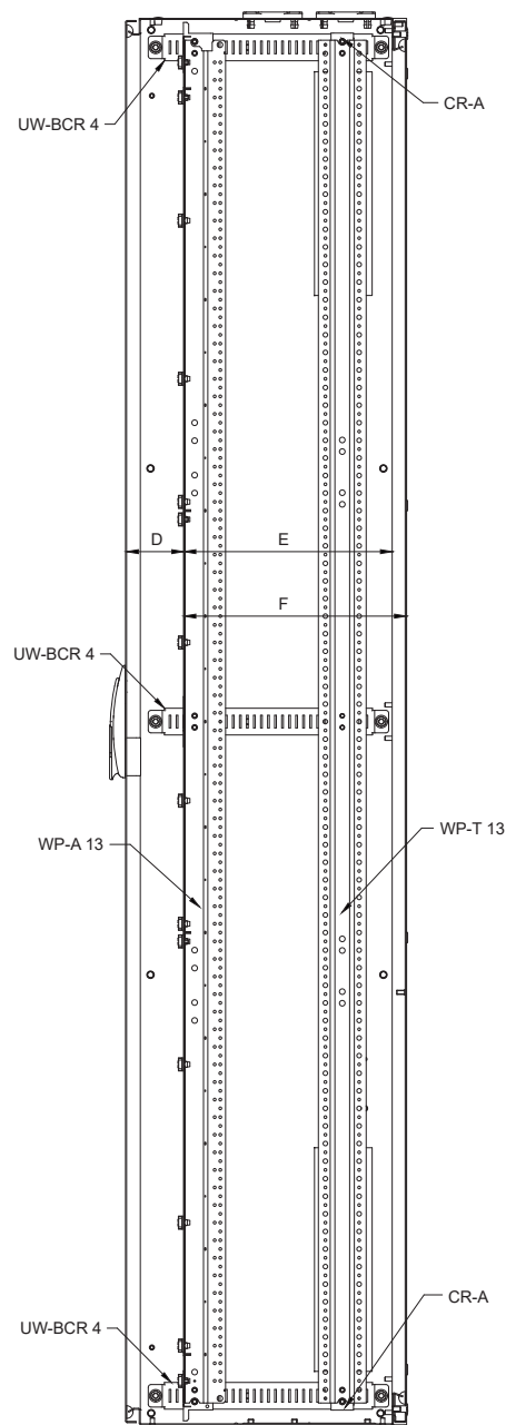
Obudowa z uchwytami UW-BCR 4 do wsporników pionowych WP-A i WP-T
