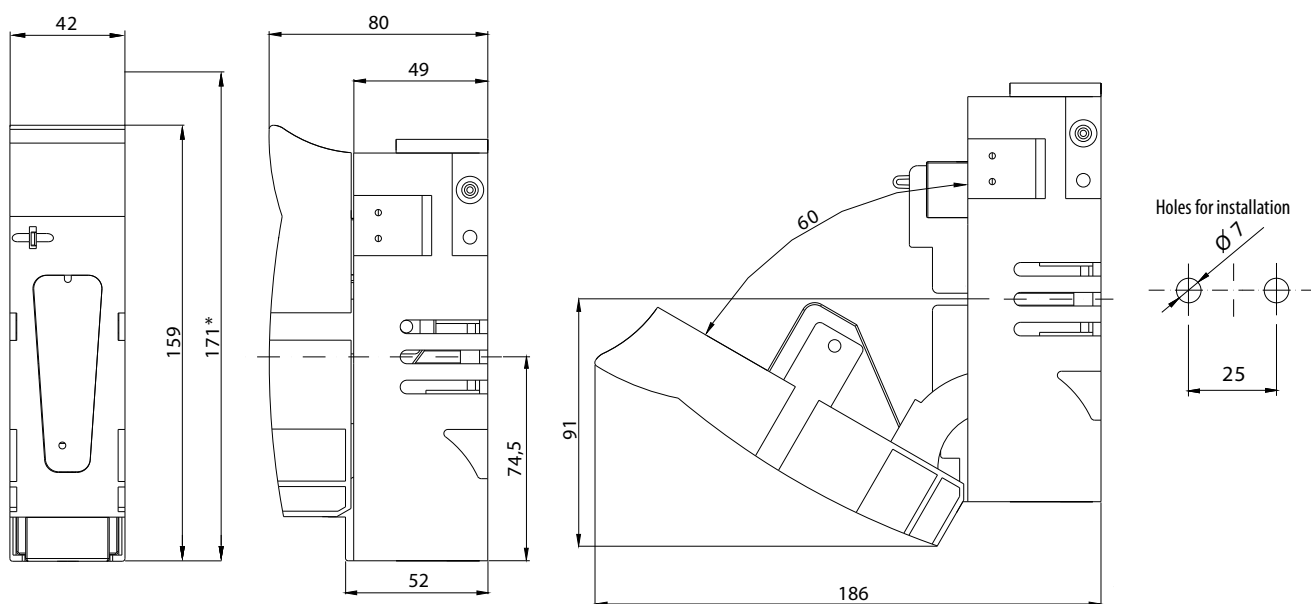
HVLEK 00 1p
