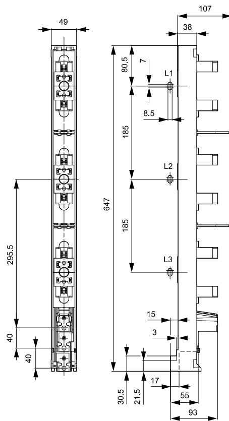
size 00/185
