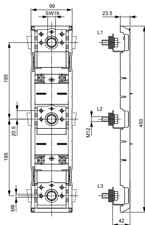
adapter DA 185-185/42
