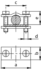
OS 00, OS 12
