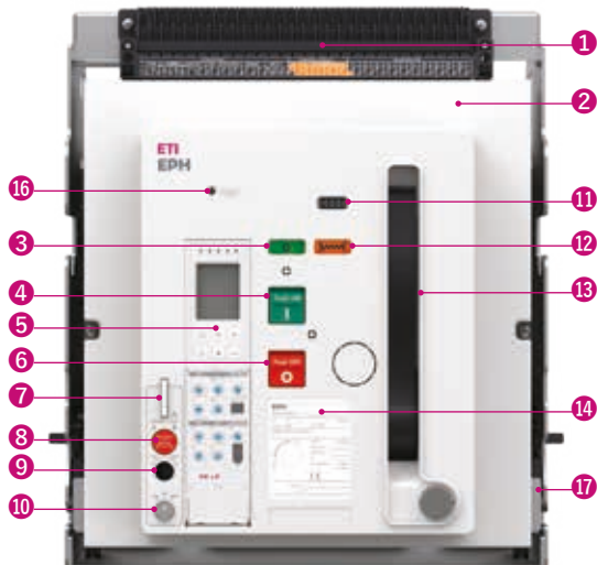
Wersja wysuwna (wyłącznik z kasetą wysuwną)
