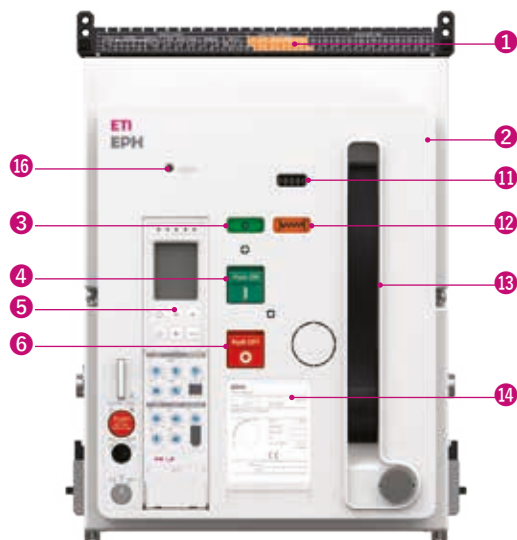
Wersja wysuwna (wyłącznik)
