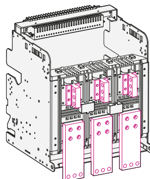
(Górne) przylłącza czołowe + (Dolne) przylłącza poziome
