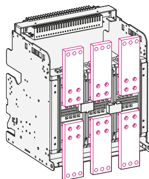
Przylłącza czołowe
