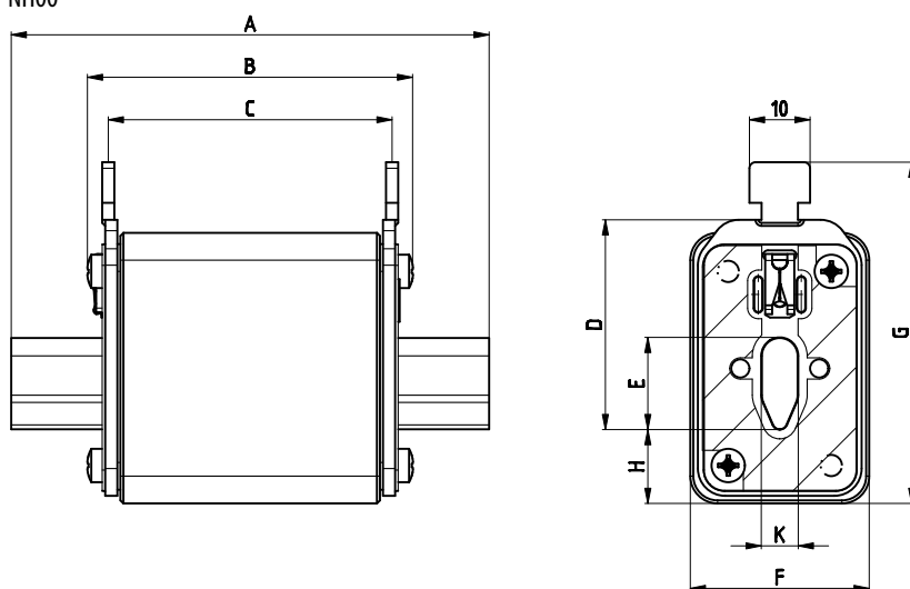
NH1, NH2, NH3 - Standard (Top) Indicator
