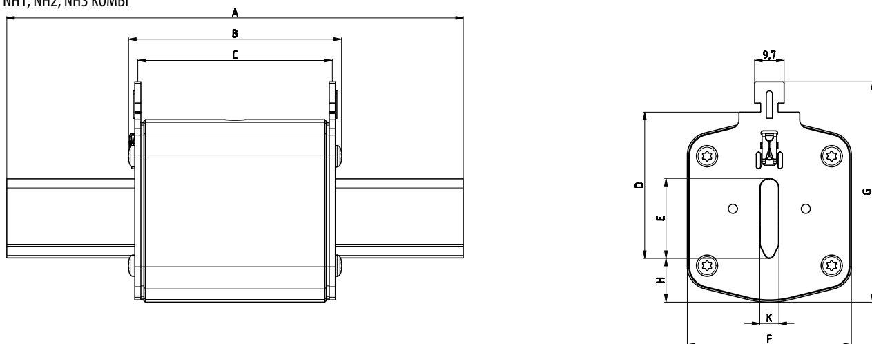
NH1, NH2, NH3 KOMBI
