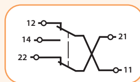
Układ styków
