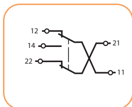
Układ styków
