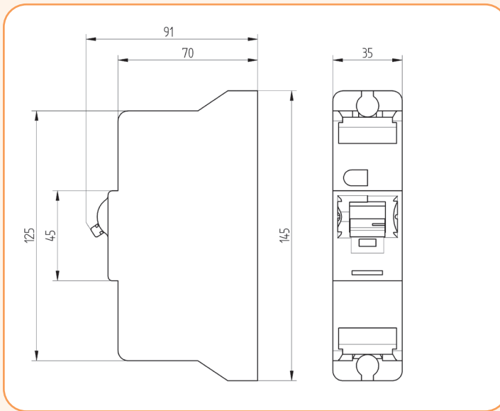
Rysunek wymiarowy
