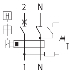
Układ połączeń-wewnętrzny
