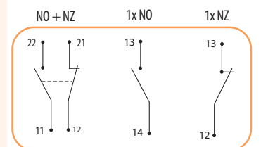
Układ styków
