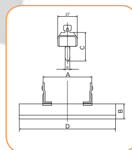
Rysunek wymiarowy
