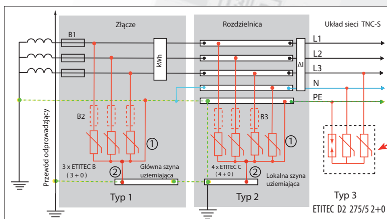
Układ połączeń ograniczników przepięć Typ1, Typ2 i Typ3 - ETITEC D2 275/5 2+0 w układzie sieci TNC-S
