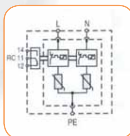
Układ wewnętrzny ogranicznika ETITEC D2 275/5 2+0
