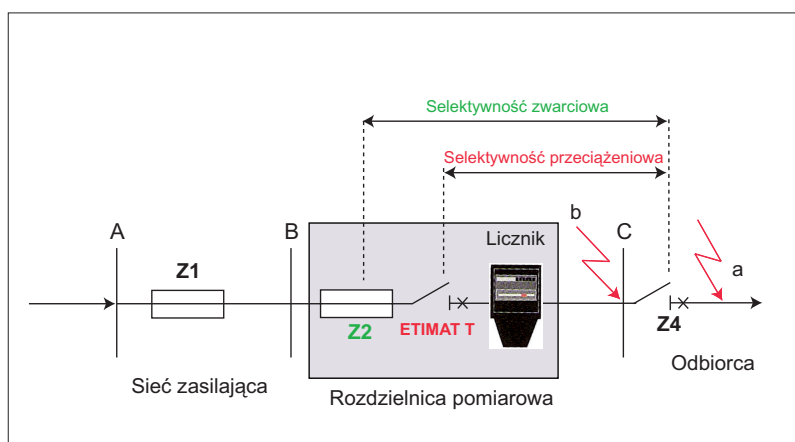
Rys. 1 Układ zabezpieczeń w tablicy licznikowej odbiorcy z wykorzystaniem ogranicznika mocy ETIMAT T
