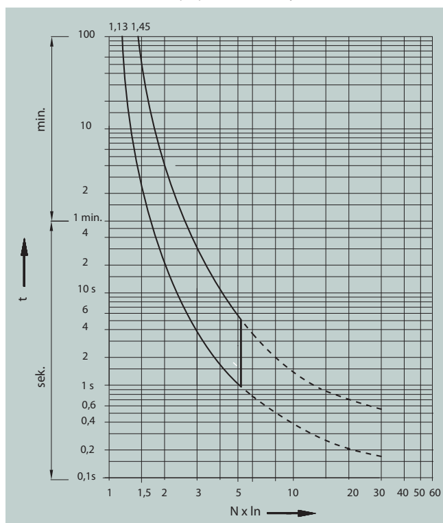
Charakterystyka czasowo-prądowa t-I
